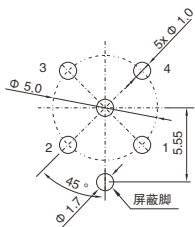
(Pin OD: \Phi 0.8) 3P/4P/5P
