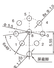
(Pin OD: \Phi 0.8) 8P
