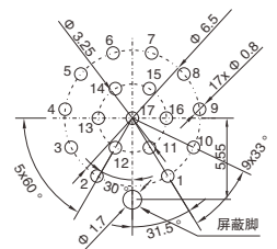
(Pin OD: \Phi 0.6) 17P
