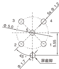
(Pin OD: \Phi 1.0) 3P/4P/5P
