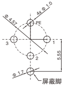
4Pin
