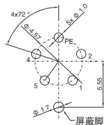
5Pin
