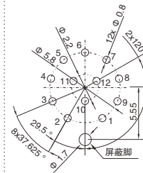
(Pin OD: \Phi 0.6) 12P
